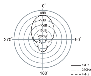
指向特性
