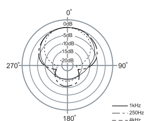
指向特性
