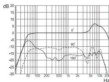
周波数特性
