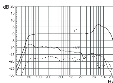
周波数特性
